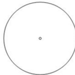
Disque de Newton en rotation Figure 2
