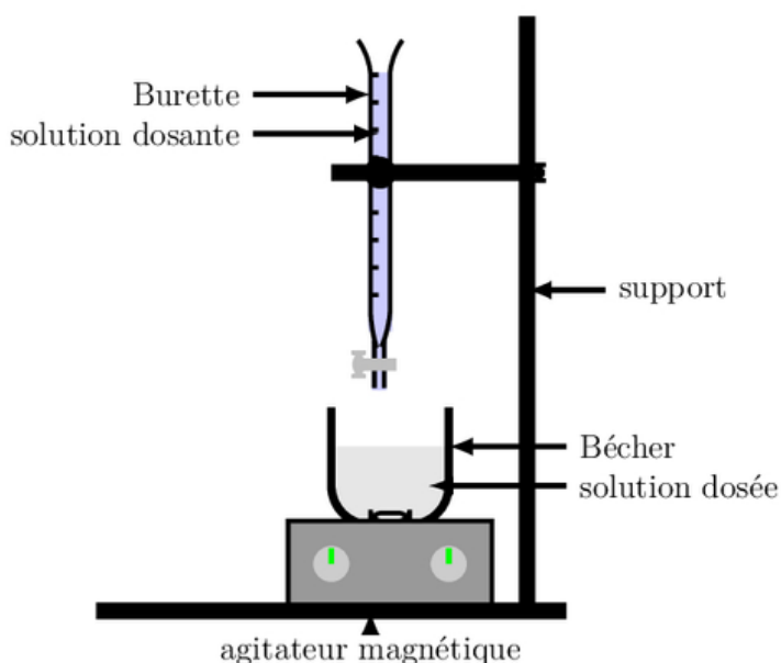
Schéma du dispositif expérimental pour un titrage
